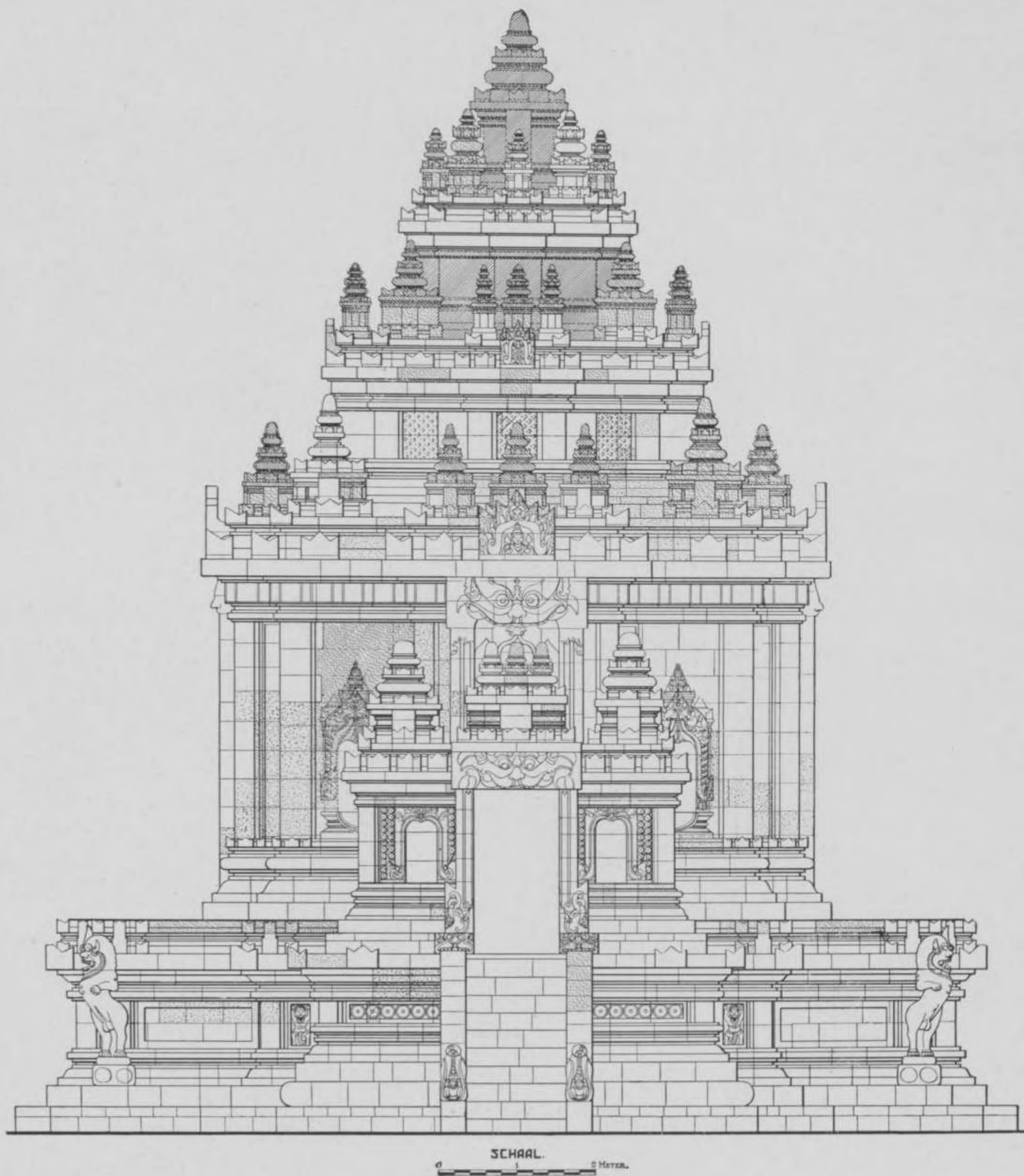
Reconstructie-teekening van den voorgevel van een der tempels te Ngawen. De gearceerde gedeelten zijn niet teruggevonden en dus niet weder opgebouwd.
